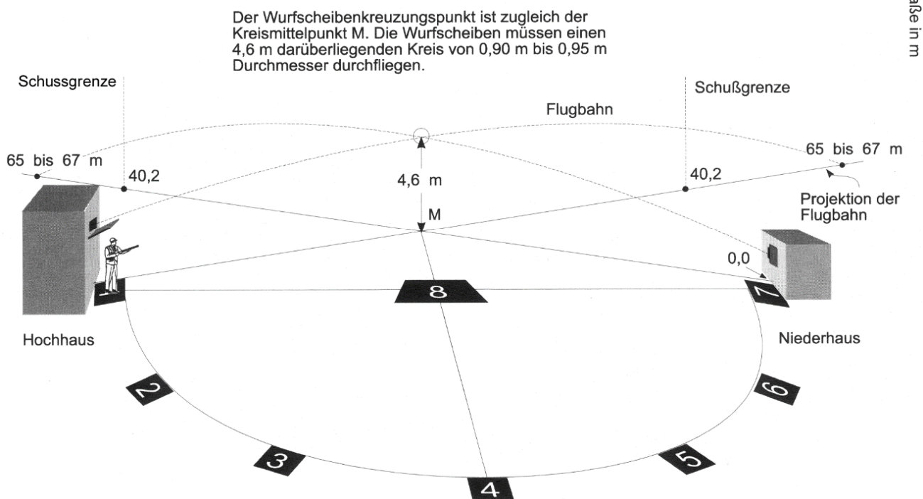
Abbildung 9.6.2.1 Wurfrichtungen und Flugweiten der Wurfscheiben beim Skeet-Schießen
