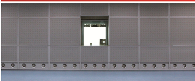
Strulik Zuluftwand SVA – eine individuelle Lösung mit garantierter Erfüllung der geforderten Strömungsparameter
