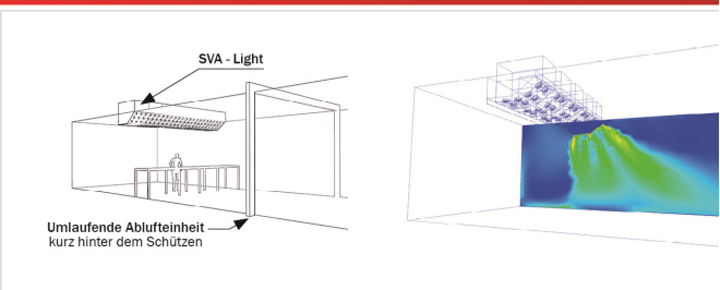
Strulik SVA-Light – Modul zur Erzeugung einer lokalen Verdrängungslüftung direkt am Schützen mit dem Hauptschützziel „Abfuhr von schädlichen Gasen vom Schützen“ (Ersparnis Volumenstrom und Gesamtinvestition-Lüftung bis zu 50 %)
