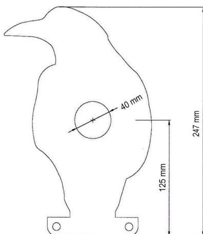
Abbildung 6.4.6.1 Beispiel einer Field-Target-Silhouette
